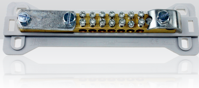
41011505 Potentialausgleichsschiene
